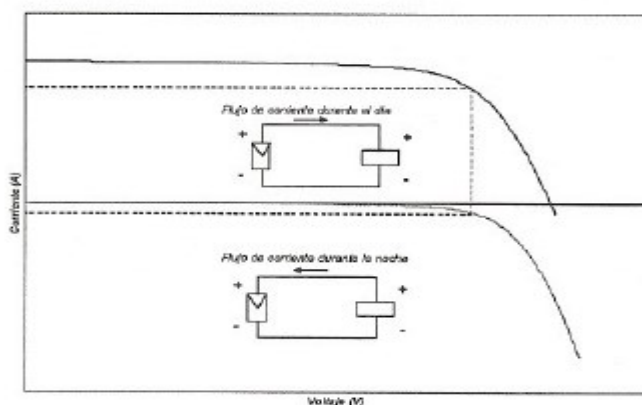
Figura: Diodos de Bloqueo
