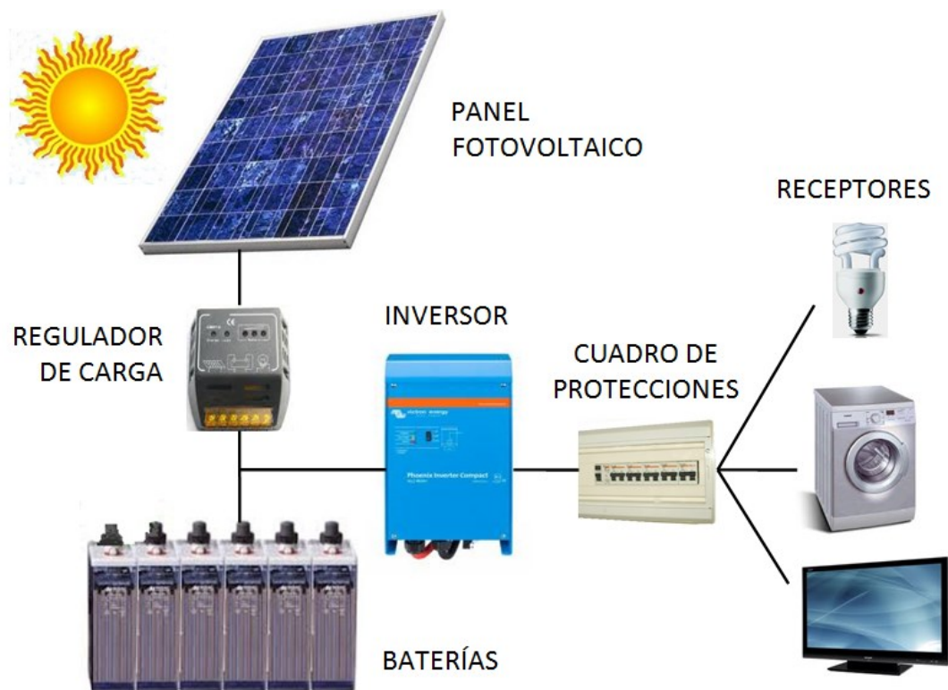
Figura 1: Diagrama físico de una Instalación Fotovoltaica
