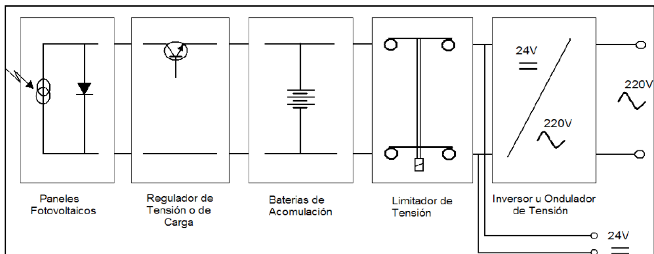
Figura 2: Diagrama eléctrico de una instalación Fotovoltaico
