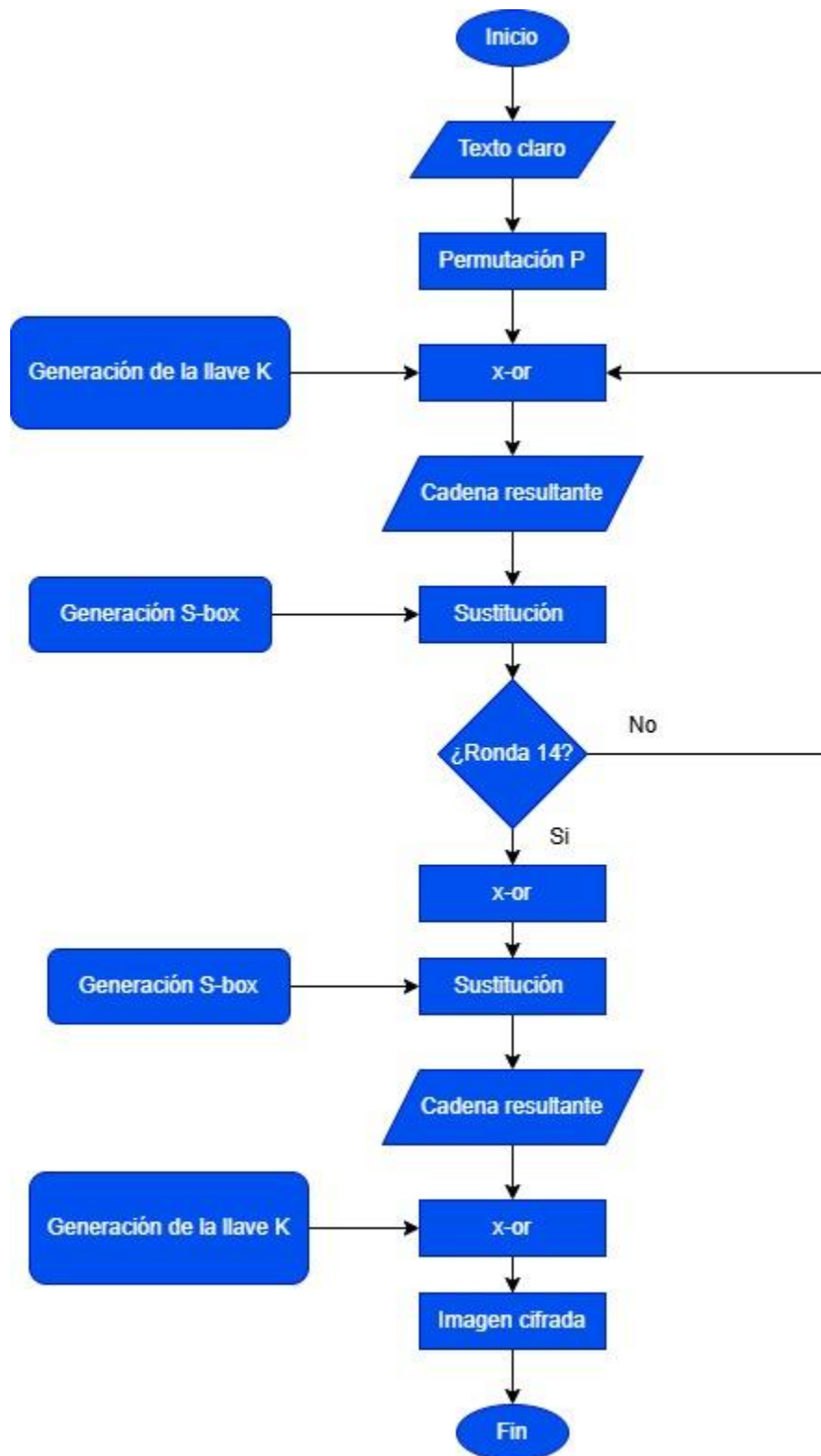
Figura 1. Proceso de Cifrado de una imagen.
