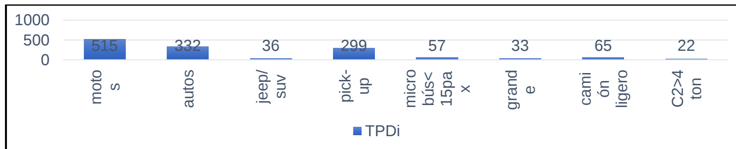
Ilustración 9. Composición vehicular estación 8+000
