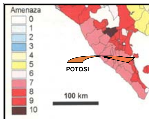
Figura N° 8. AMENAZA POR SISMICIDAD.
