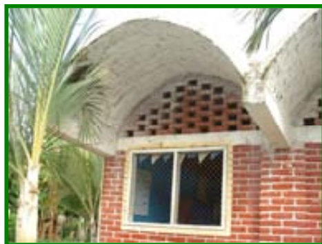
Detalle de la Bóveda Autoportante
